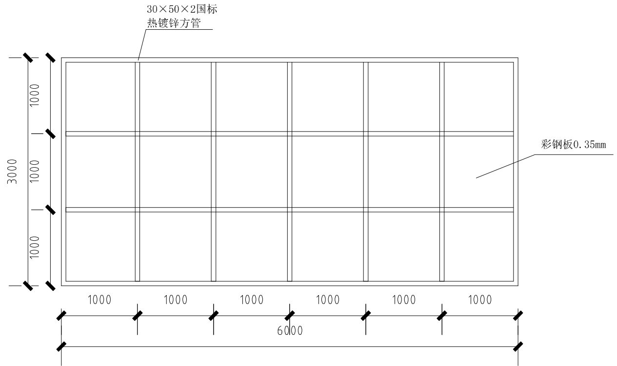
立面图
