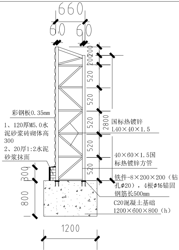
立柱及基础详图 立柱间距3000mm
