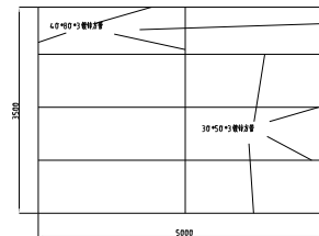
三视图立面图
