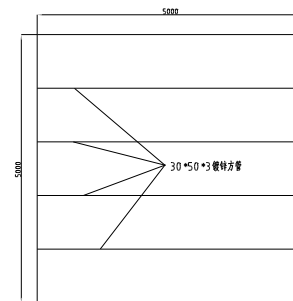
平面图
